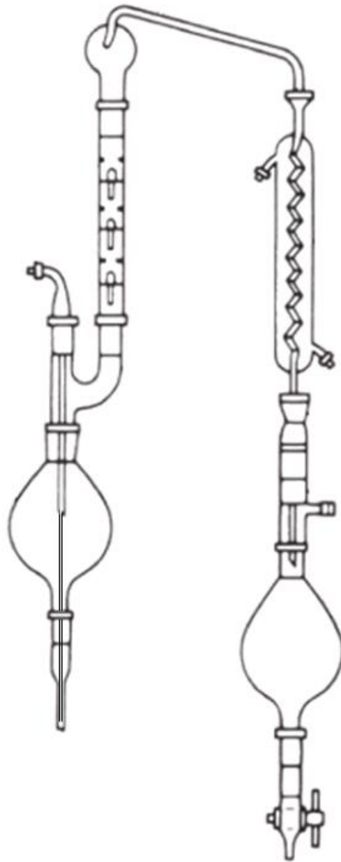
図 5 クデルナダニッシュ型濃縮器
