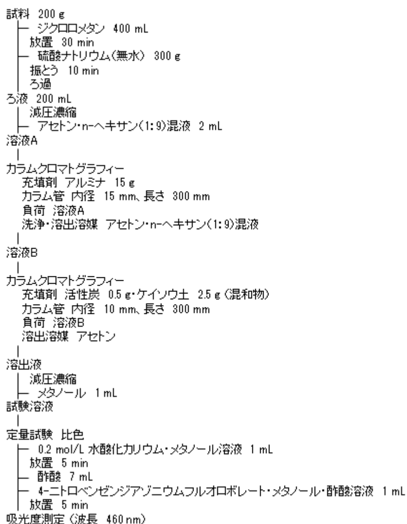
図 3 昭和 47 年 5 月 31 日厚生省告示第 177 号で提示されたカルバメイト剤試験法
