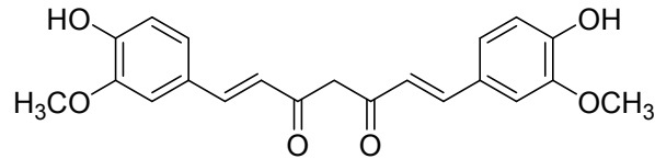
クルクミン
