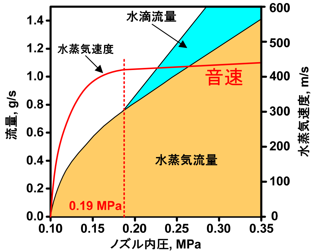
図4 アクアガス/過熱水蒸気の発生条件 —水蒸気流量、水滴流量とノズル内圧の関係—
