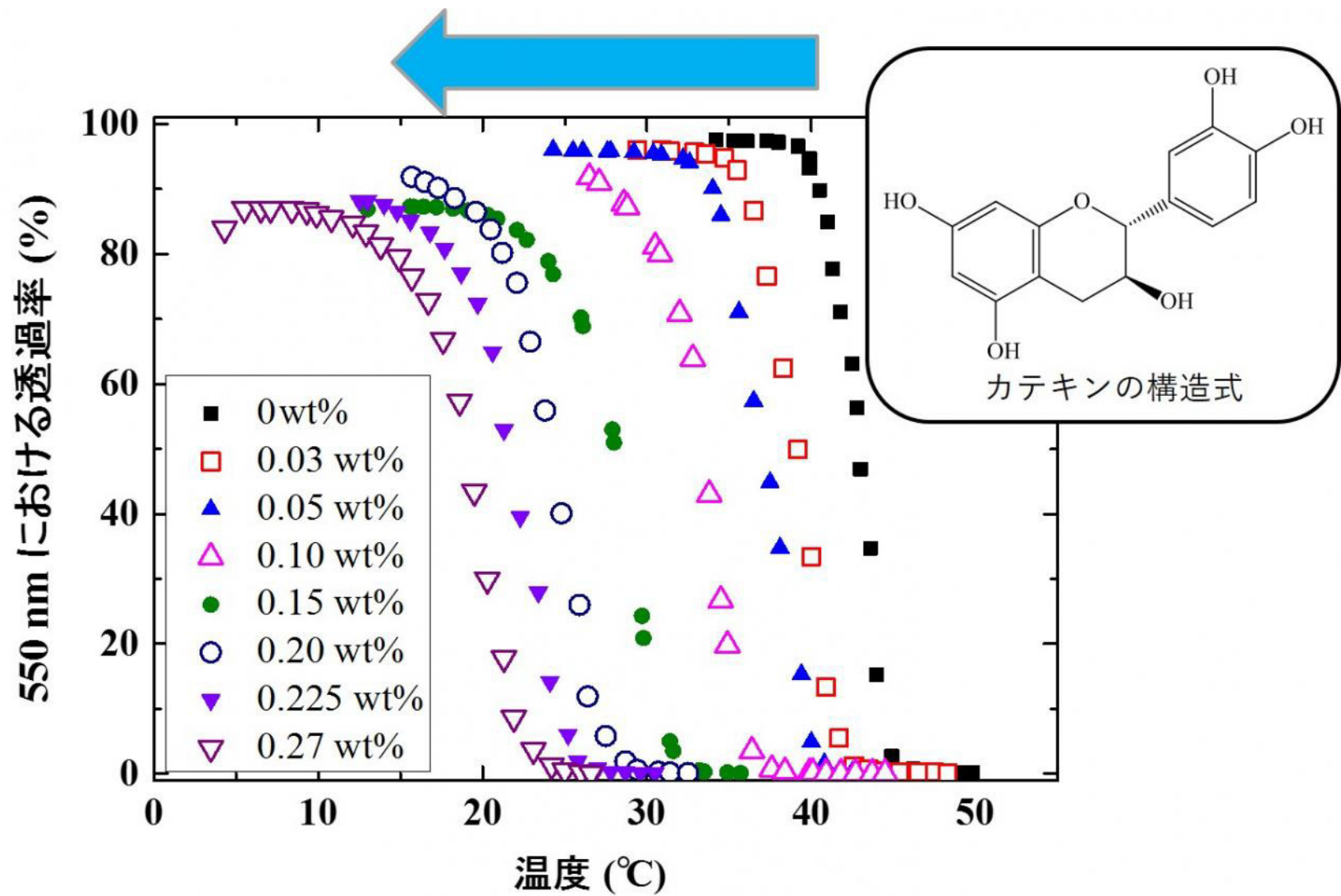
図4 カテキン添加濃度がHPCの相転移挙動に及ぼす影響
