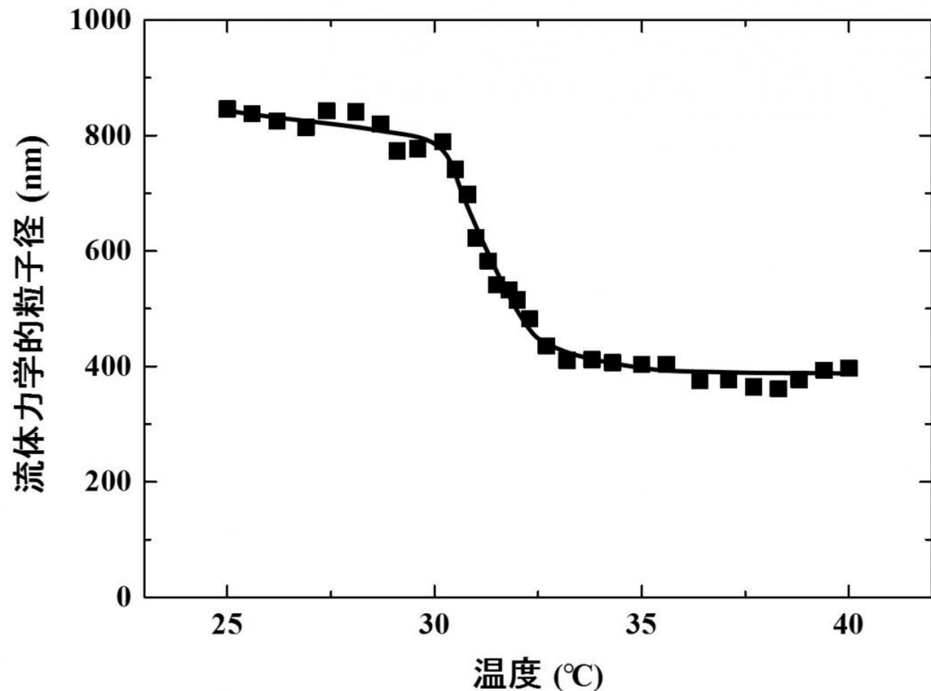
図3 PNIPAMジェル粒子の水中粒子径に及ぼす温度の影響
