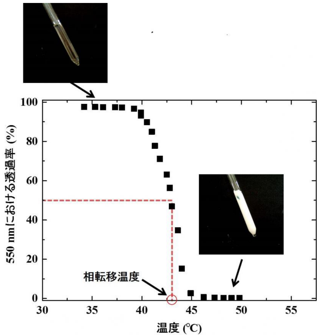
図1 ヒドロキシプロピルセルロースの透過率-温度曲線
