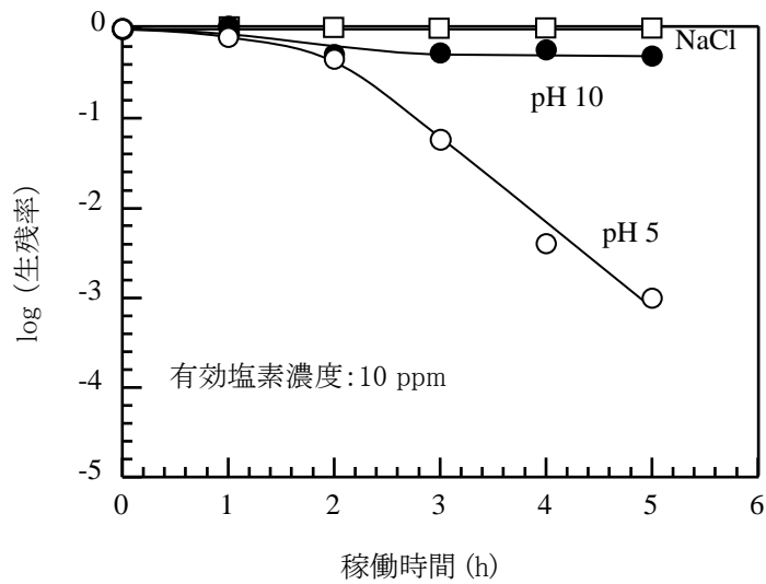
図7. NaCl 水溶液 および NaOCl 水溶液を供給した通風気化装置を稼働したときの湿潤ガーゼ付着菌に対する吹き出し空気の殺菌効果
