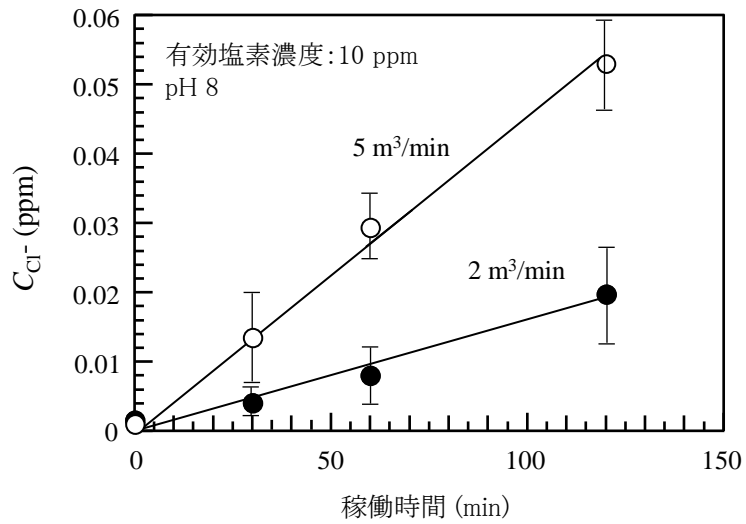
図6. NaOCl水溶液を供給した通風気化装置を異なる風速で稼働したときの C_{Cl^-}
