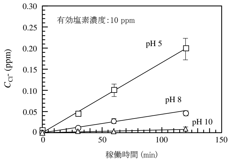
図4. pHの異なるNaOCl水溶液を供給した通風気化装置を稼働したときの C_{Cl^-}
