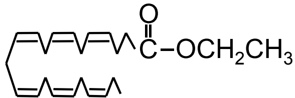
DHAエチル (エチルエステル(EE)形態)
