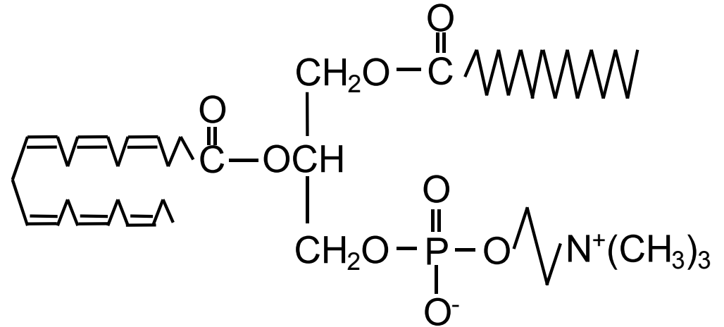
sn -2 DHA-ホスファチジルコリン (リン脂質(PL)形態)
