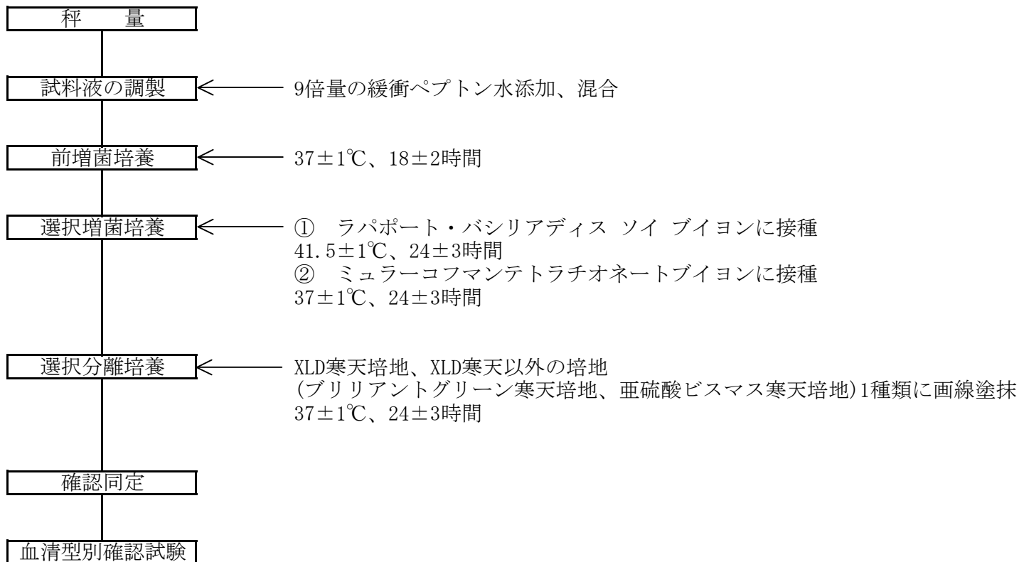
図-2 ISO 6579 : 2002(E) の検査法
