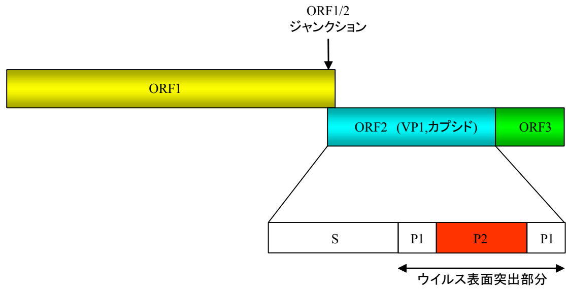
図4 ゲノム構造模式図
