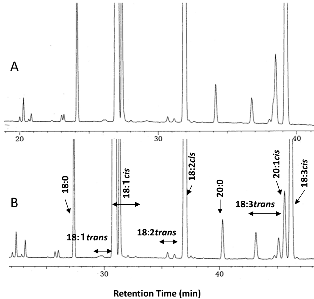
図8. カラムEを用いて、カラム温度を180°C(A)と175°C(B)で測定したときの キャノーラ油のガスクロマトグラフィー
