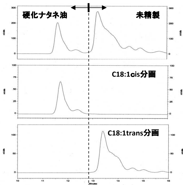
部分水素添加ナタネ油のC18:1異性体のHPLCによる分離
