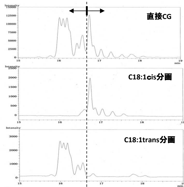
直接GC分析と逆相HPLC法で分離した各分画のGC分析
