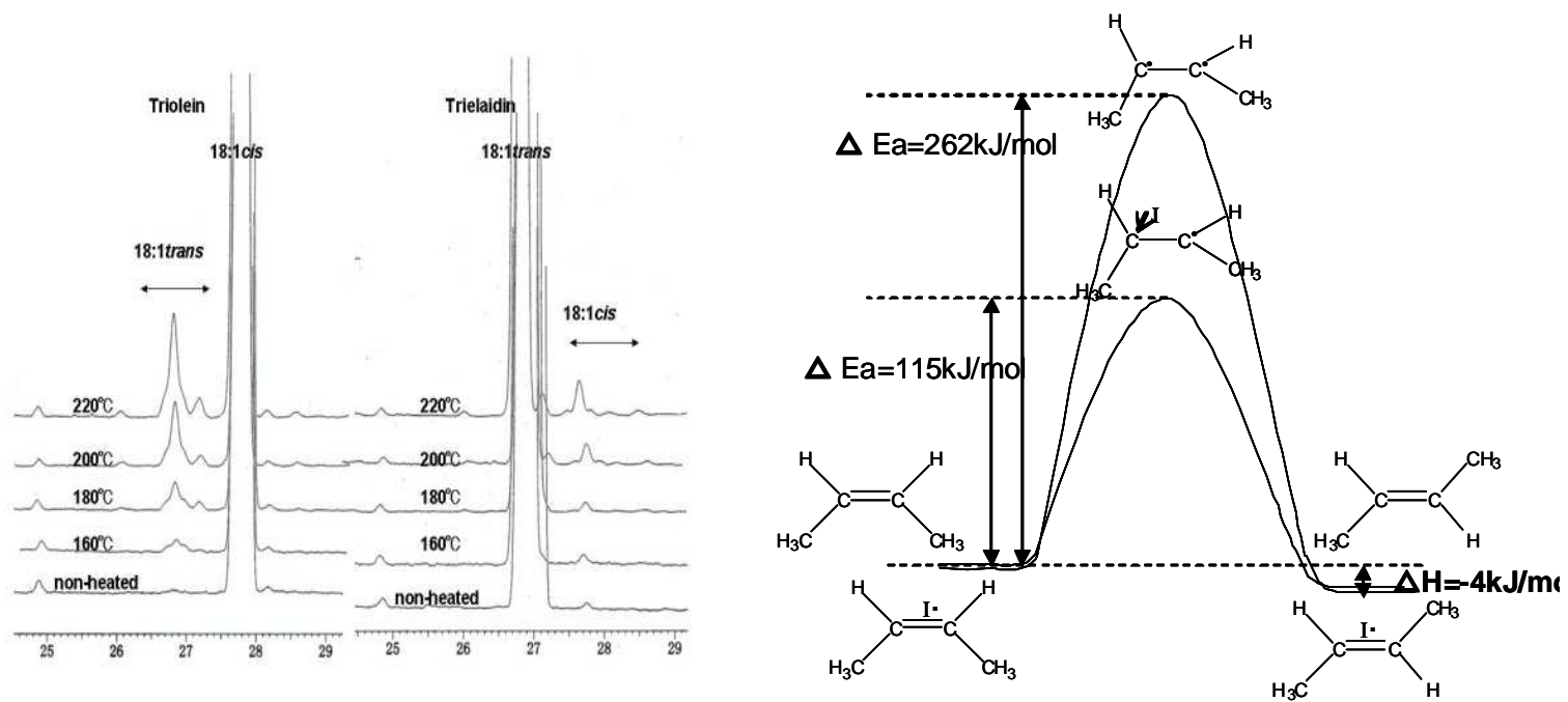
図5. (A)トリオレイン( cis 9,18:1、左)とトリエライジン( trans 9,18:1、右)を各温度で連続加熱したときの異性化と (B)アレニウスプロットより算出されたラジカル脂質の二重結合の活性化エネルギー
