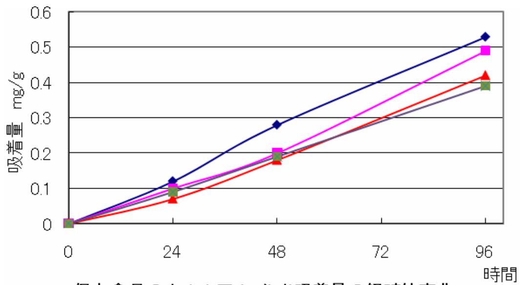
Fig. 3 保存食品のホルムアルデヒド吸着量の経時的変化 at20°C
