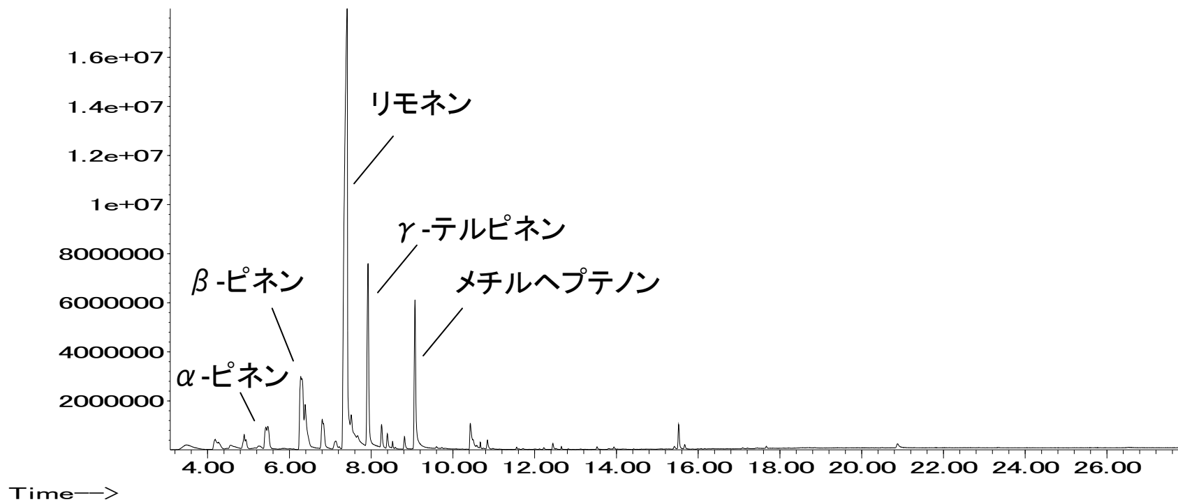
図2.透過確認試験に用いた牛乳のクロマトグラム
