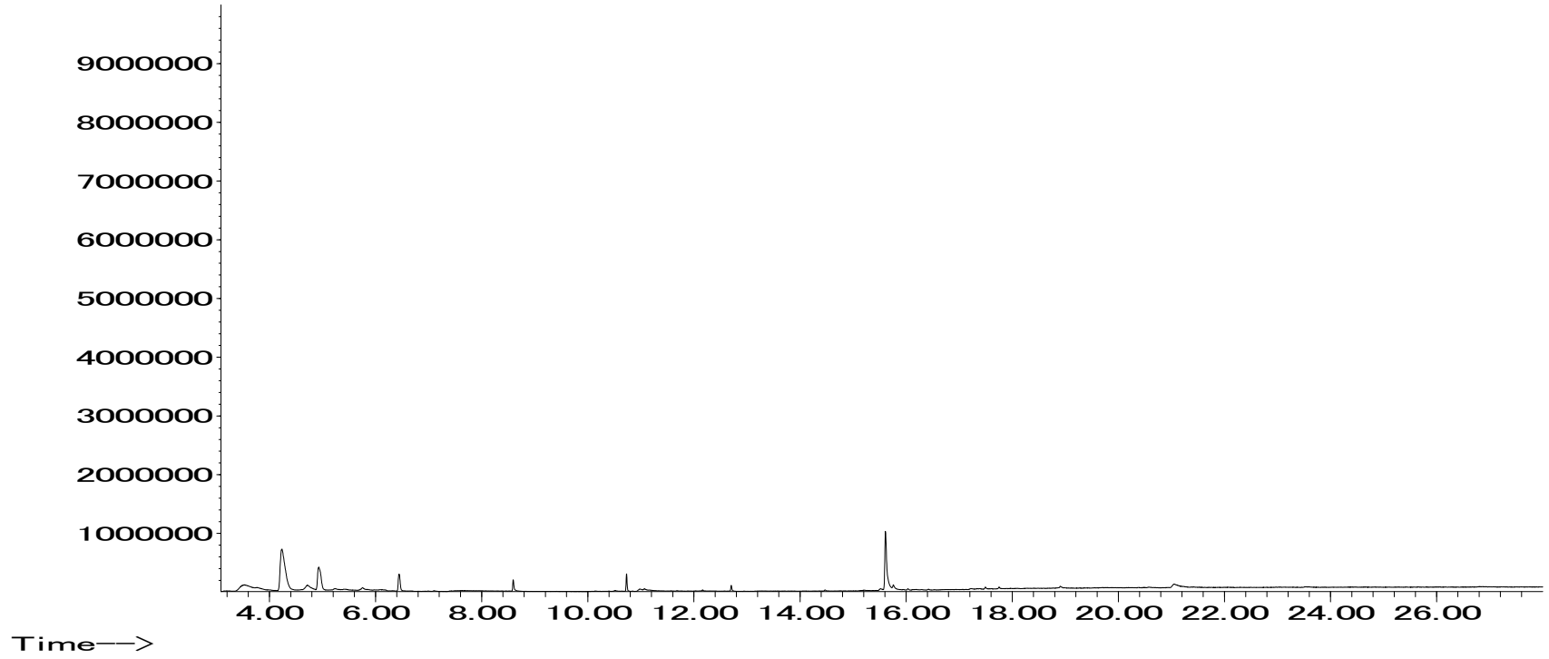
図1.牛乳のクロマトグラム
